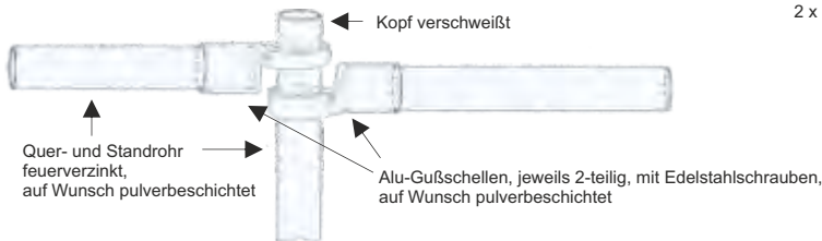
Montagebeispiel starres Geländer
