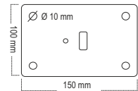
Fußplatte für klappbare Poller 8 mm dick
