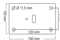
Fußplatte für Poller Ø 60-89 mm 8 mm dick
