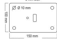
Fußplatte für klappbare Poller 8 mm dick
