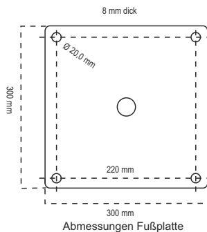
Abmessungen Fußplatte
