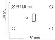
Fußplatte für Poller Ø 60-89 mm 8 mm dick
