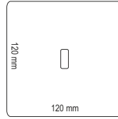
Fußplatte für klappbare Poller 6 mm dick
