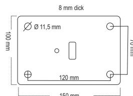
Abmessung der Fußplatte für Pfosten 70x70, Ø 76 und 89 mm
