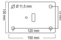
Fußplatte für Poller Ø 60-89 mm 8 mm dick
