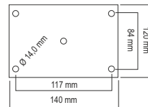
Fußplatte für Poller ab Ø 102 mm 8 mm dick
