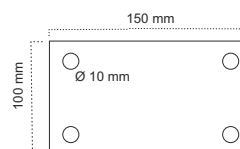
Bedarfsweise Fußplatten 100 x 150 x 8 mm
