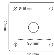
Fußplatte für klappbare Poller 8 mm dick
