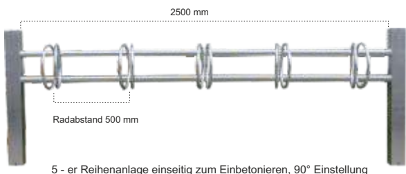
5 - er Reihenanlage einseitig zum Einbetonieren, 90° Einstellung
