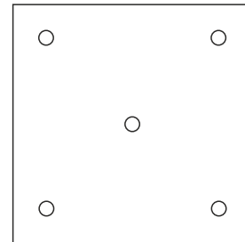
Fußplatte 200 x 200 x 8 mm Lochbohrung Ø 20 mm Lochmitte / Lochmitte 160 mm
