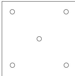
Fußplatte 300 x 300 x 10 mm Lochbohrung Ø 20 mm Lochmitte / Lochmitte 220 mm
