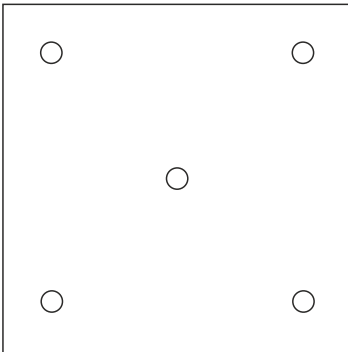
Fußplatte 360 x 360 x 8 mm Lochbohrung Ø 22 mm Lochmitte / Lochmitte 260 mm
