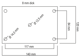
Fußplatten - Abmessung für Pfosten Ø 102 mm
