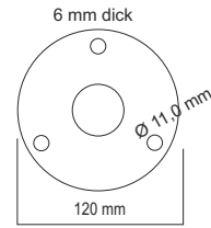
techn. Daten der Fußplatte für Pfosten Ø 48 mm und Ø 60 mm
