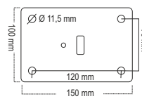
Fußplatte für Poller Ø 60-89 mm 8 mm dick
