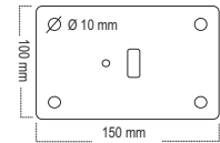
Fußplatte für klappbare Poller 8 mm dick
