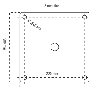
Abmessungen Fußplatte
